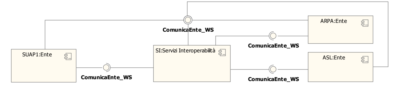
Figura 19. Architettura logica: interfacce a supporto dello scenario 2 (interazione SUAP – Enti)
