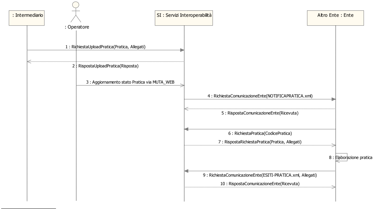
Figura 18. Scenario 1: esempio di interazioni
