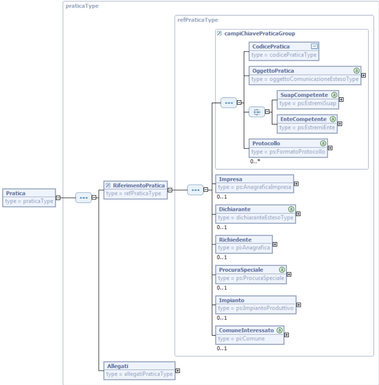
Figura 2. Struttura dell'elemento <Pratica>
