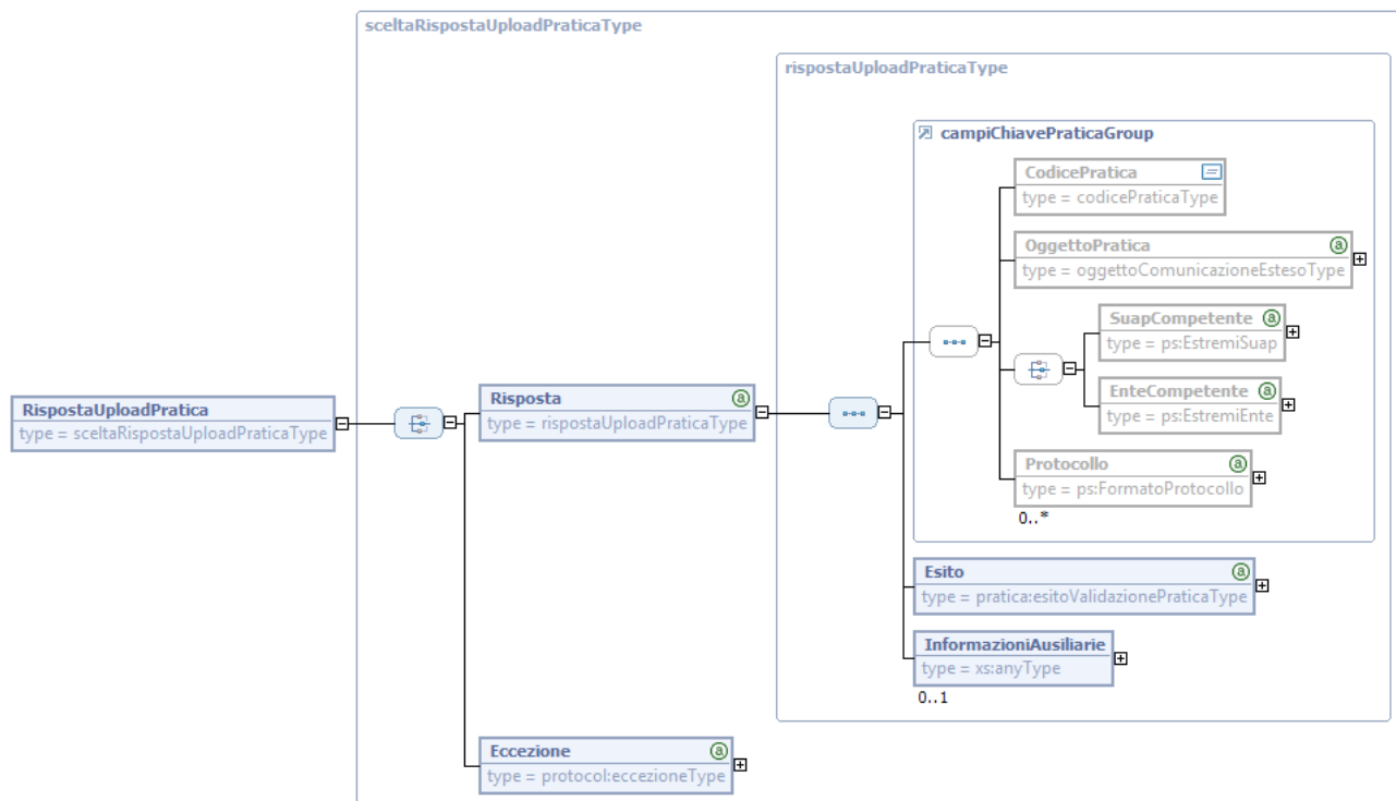
Figura 7. Struttura dell'elemento <RispostaUploadPratica>
