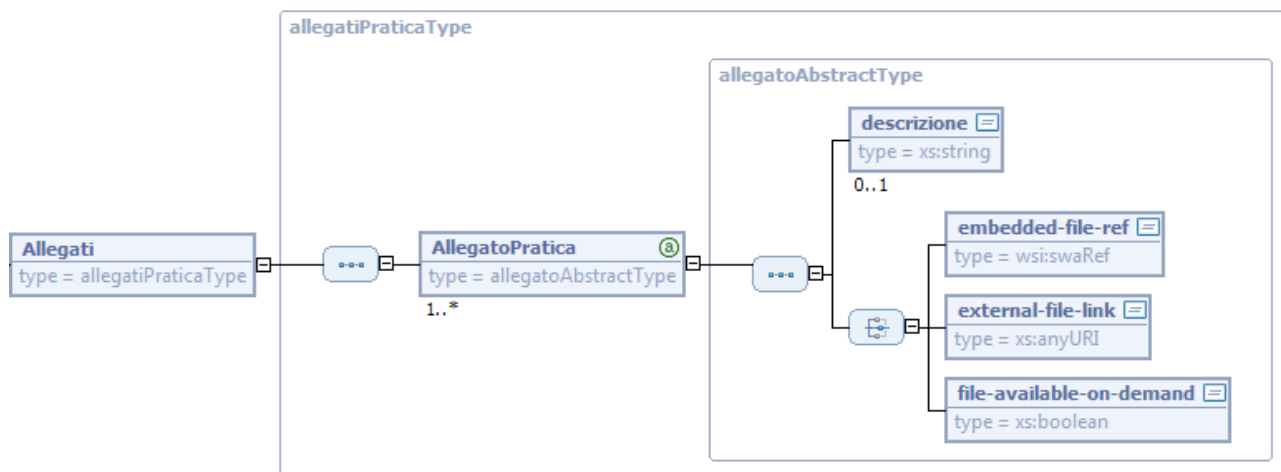
Figura 3. Struttura dell'elemento <Allegati>
